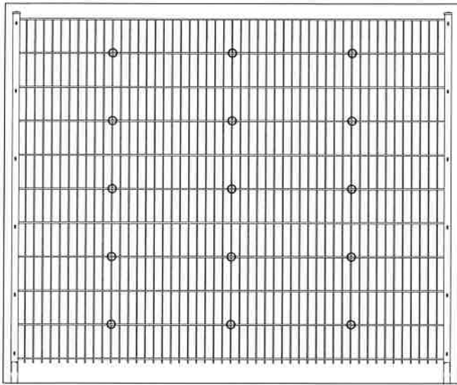
Beispiel Platzierung der Schraubspanner bei Höhe der Steinmauer von 2000 mm
